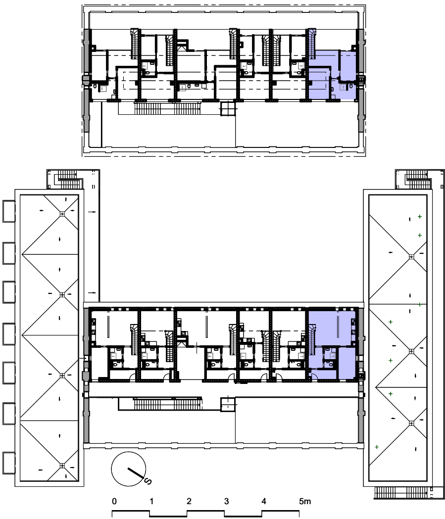
Schéma půdorys
